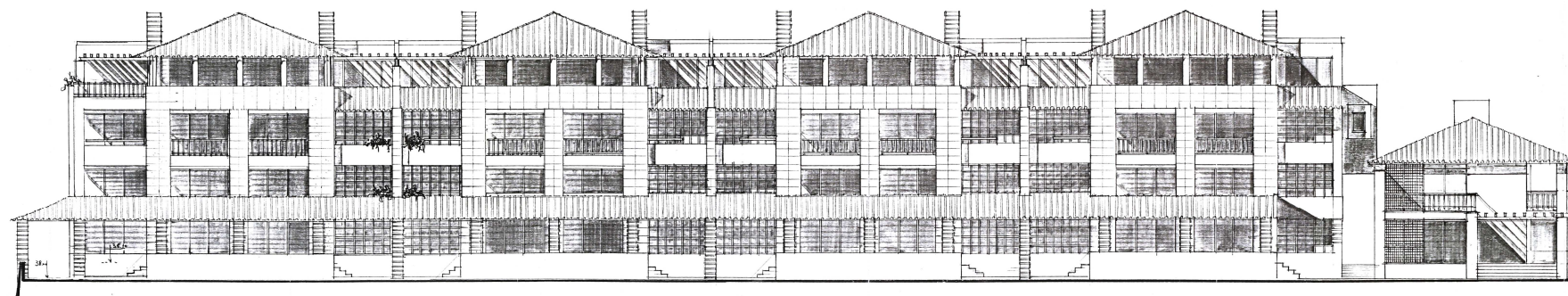
Alçado Sul
